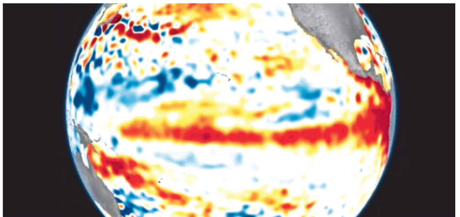
EXPECTATIVA É QUE HAJA AUMENTO NO NÍVEL DO MAR NAS REGIÕES DAS BANHADAS PELAS ÁGUAS DO OCEANO PACÍFICO EQUATORIAL
